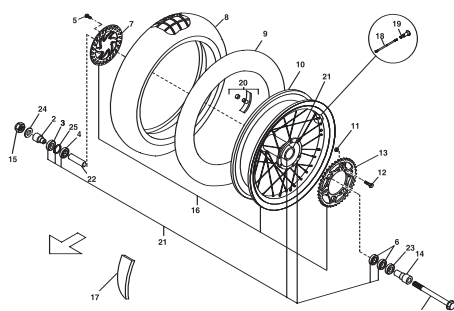
TAV.29 Ruota posteriore - Rear wheel - Roue AR. - Hinterrad - Rueda trasera
