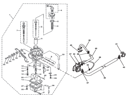
TAV.7 Carburatore - Carburettor - Carburateur - Vergaser - Carburador
