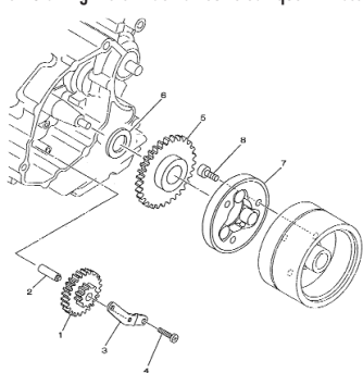
TAV.13 Ingranaggi Cambio - Gear group - Engrenages changement de vitesses - Schaltgetriebe - Engranaje del cambio
