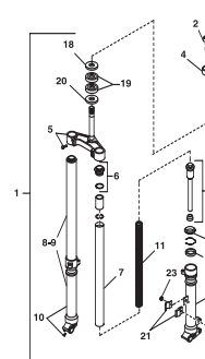
TAV.22 Forcella anteriore - Front fork - Fourche AV. - Vorderradgabel - Horquilla delantera
