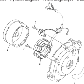
TAV.18 Dispositivi elettrici - Electrical devices - Dispositifs electriques - Elektrische Ausrüstung - Dispositivos electricos
