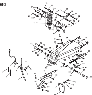
TAV.21 Sospensione posteriore - Rear suspension - Suspension AR. - Hintere aufhängung - Suspensión trasera
