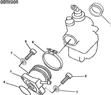
TAV.6 Raccordo d'ammissione - Induction pipe - Raccord d'admission - Ansaugstutzen - Racor de admision
