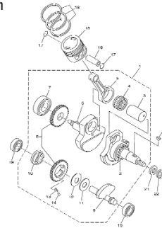
TAV.2 Albero motore-Piston - Crankshaft-Piston - Vilebrequin-Piston - Kurbelwelle-Kolben - Cigüeñal-Pistón
