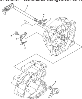
TAV.17 Motorino avviamento - Starting motor - demarreur electrique - Anlassermotor - Motor de arranque
